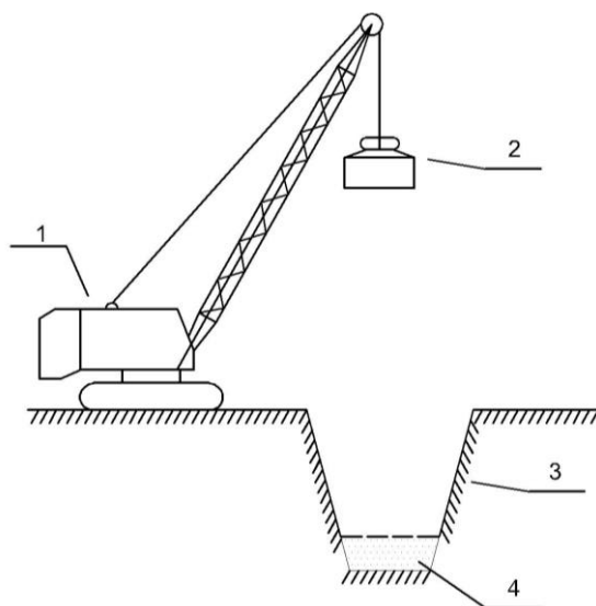
Рисунок 1 – Уплотнение основания шурфа (траншеи)
