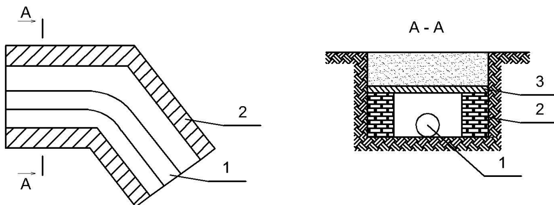
Рисунок 3 – Устройство непроходного канала
